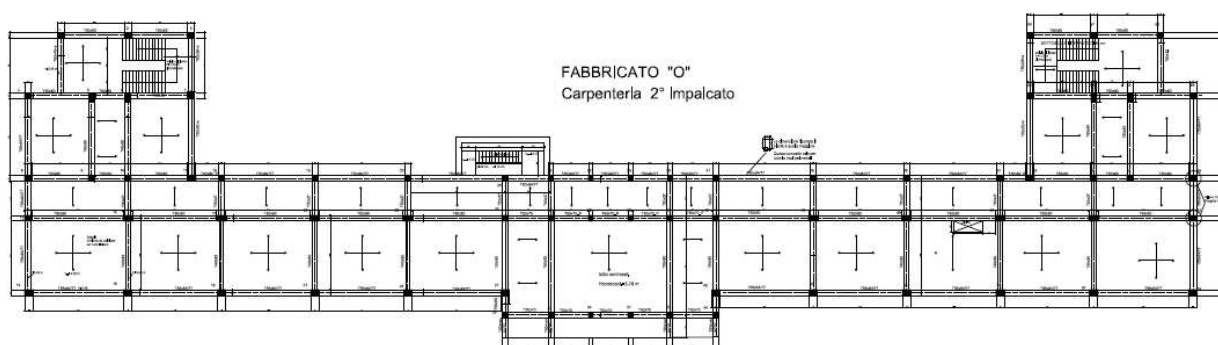
Fig. 2: Edificio O, Carpenteria impalcato tipo
